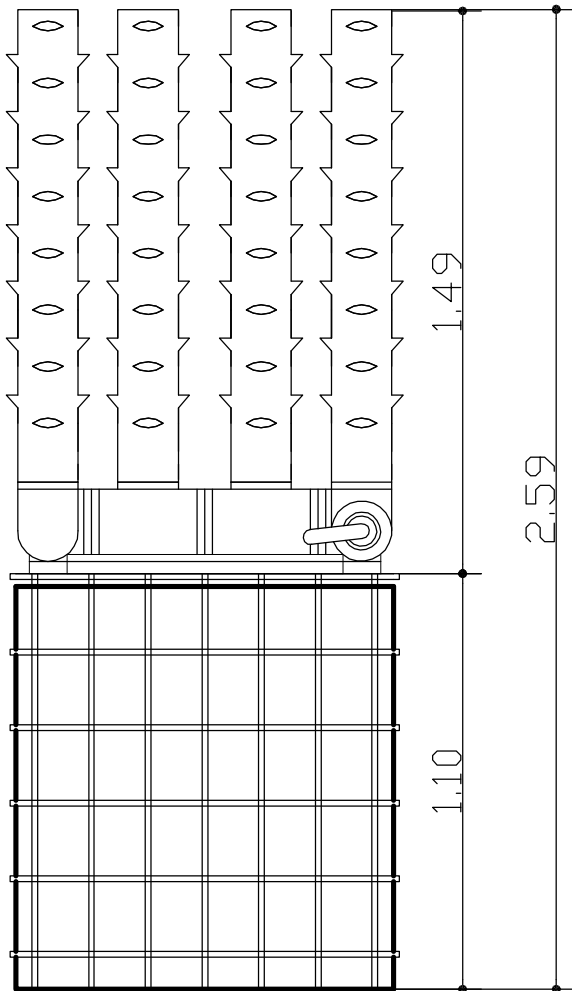
ALZADO
